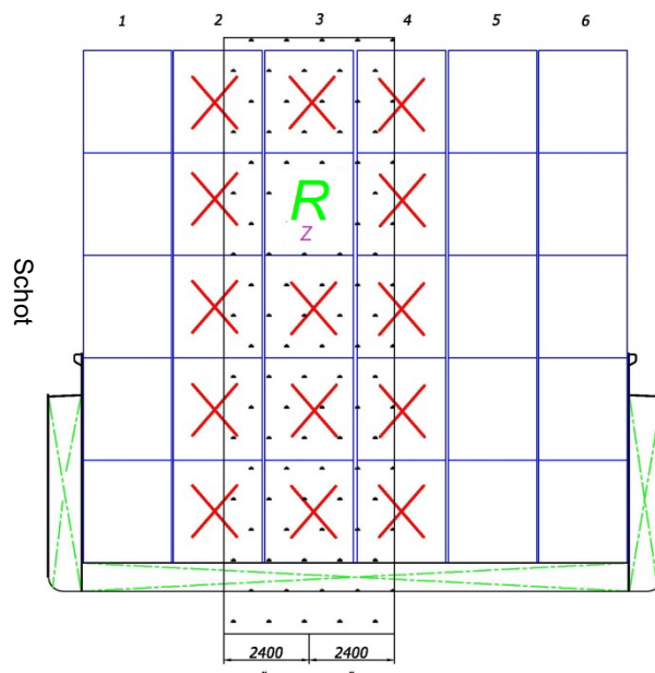
Vooranzicht
